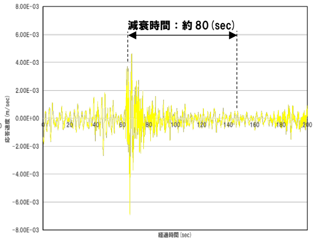
(c) 3回目ねじれ方向衝撃振動波形
