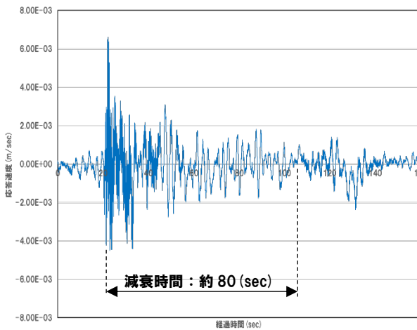
(b) 2回目ねじれ方向衝撃振動波形
