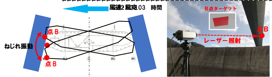
(b) 風によるねじれ振動
