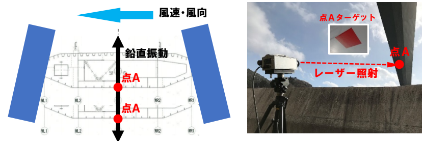
(a) 風による鉛直振動
